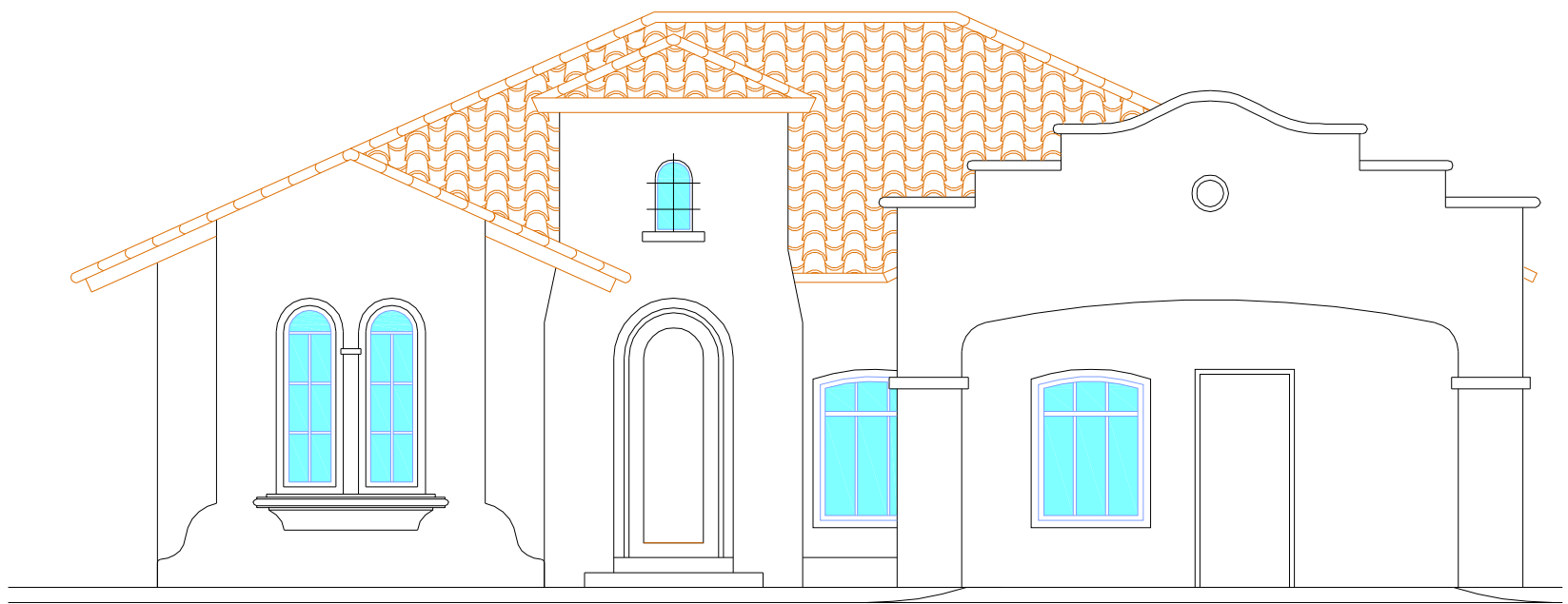
FACHADA FRONTAL MODELO "A"
